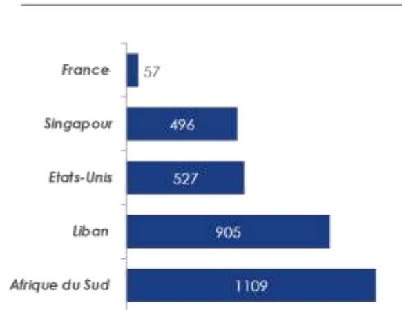
Intensité carbone de l'électricité par pays (en gCO 2 e/kWh)
