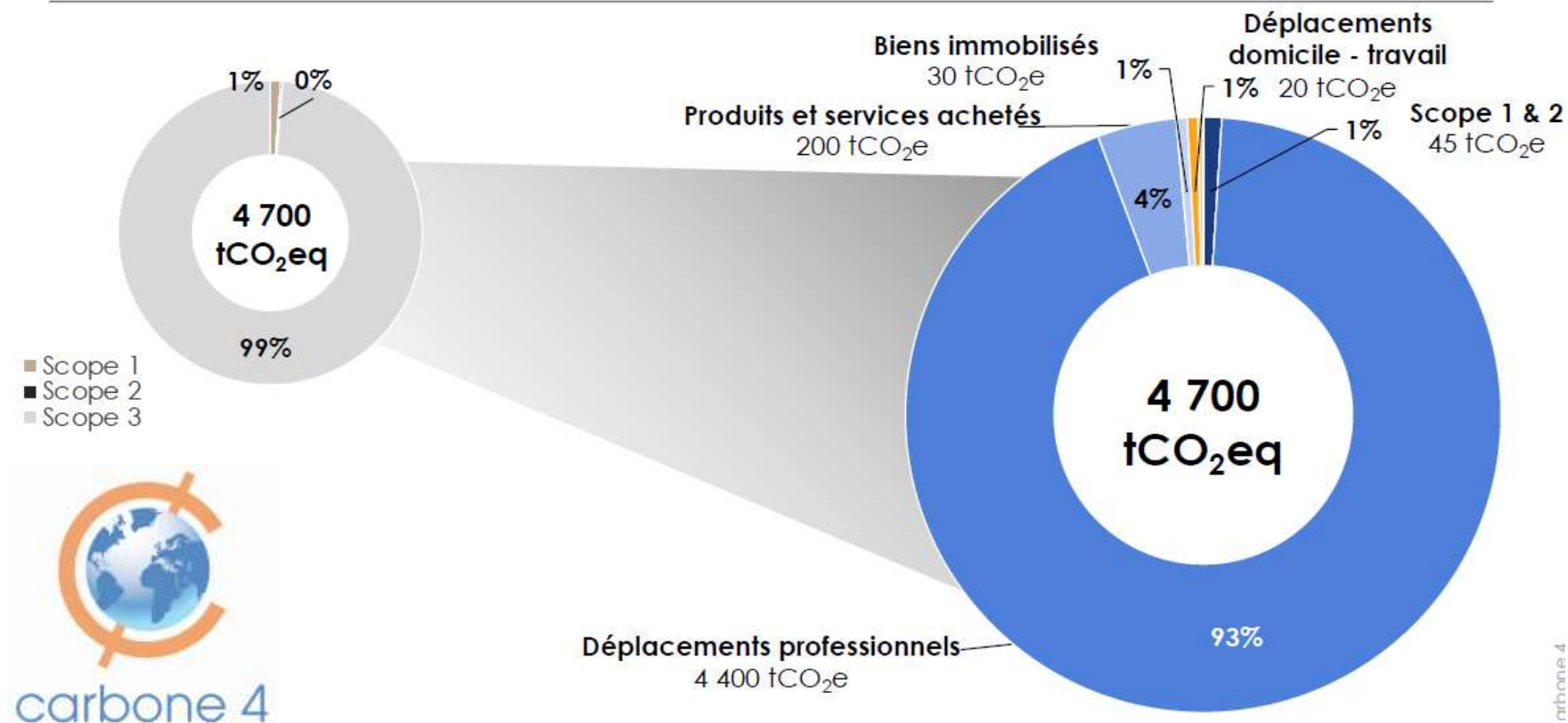
Émissions de CO 2 e par scope et détail du scope 3 (tCO 2 e, % des émissions totales)
