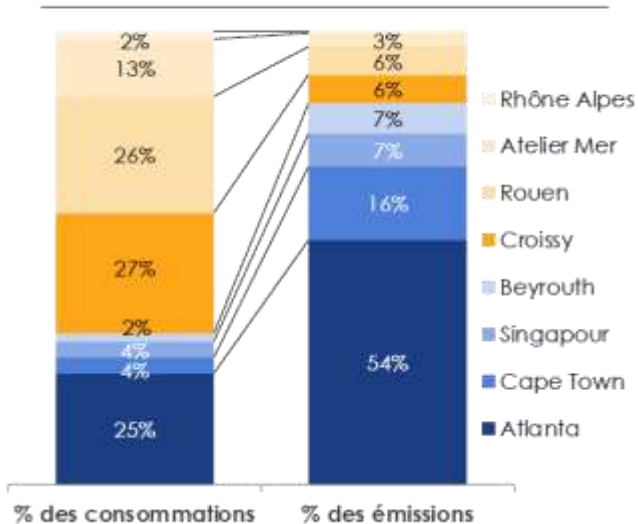
Répartition des émissions et des consommations d'électricité (%)
